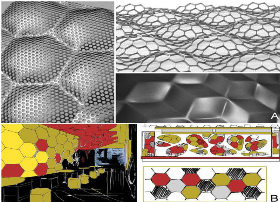
نمودار ۴. سازه‌های لانه زنبوری فنی برای استفاده در معماری. دکتر Mirtsch GmbH، با مجوز از Frank Mirtsch. و کندو، معماری داخلی با الهام از حشرات طراحی شده توسط Kyle Minnock، لیدز، انگلستان؛ ماخذ: یافته‌های تحقیق.
