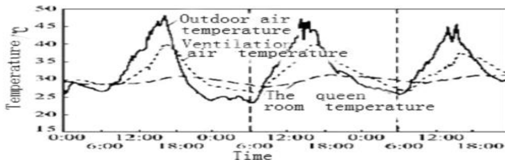
شکل ۳. اختلاف دما در لانه (تپه) موربانه؛ ماخذ: Zari MP 2019
