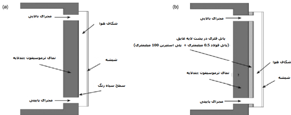
شکل ۱۳. دیاگرام شماتیک سیستم‌های دیوار ترومب الف) دیوار ترومب کلاسیک ب) دیوار ترومب بهبود یافته
