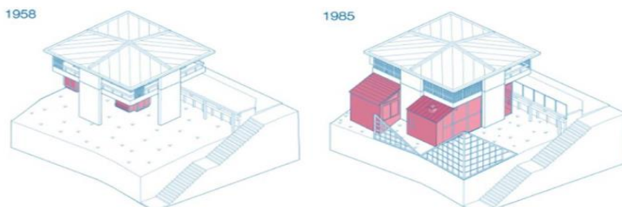
شکل ۶. ساختمان اسکای هاوس که کیمونو کیکوتاکه طراحی کرده است: الف) اسکای هاوس در سال ۱۹۵۸، ب) اسکای هاوس در سال ۱۹۸۵؛ ماخذ: Sherman BD, 2014، جدول ۳. تحلیل نمونه‌های بیونیک سازه ساختمانی؛ ماخذ: نگارندگان.
